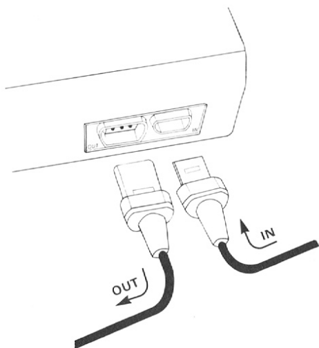
Figure 1-1 HP-IL Cables
